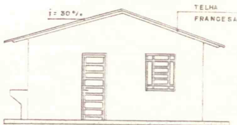
ELEVAÇÃO FRONTAL E1
